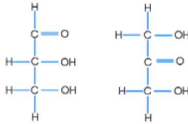
D-Gliceraldehído (aldosa)
